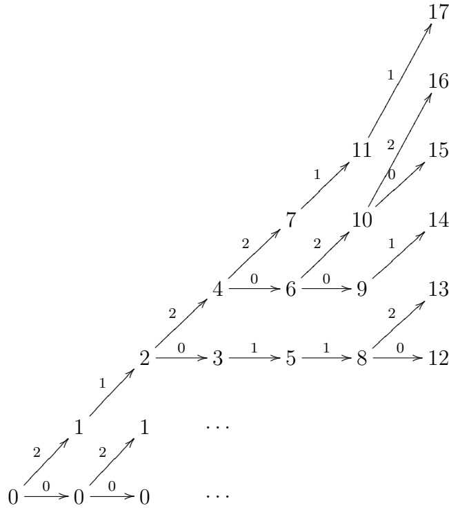
図 1: 3/2 数系の Tree
